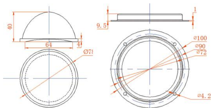
чертёж линзы
