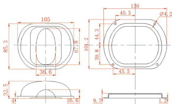
чертёж линзы
