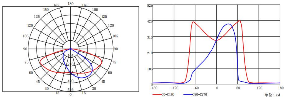
配光曲线
