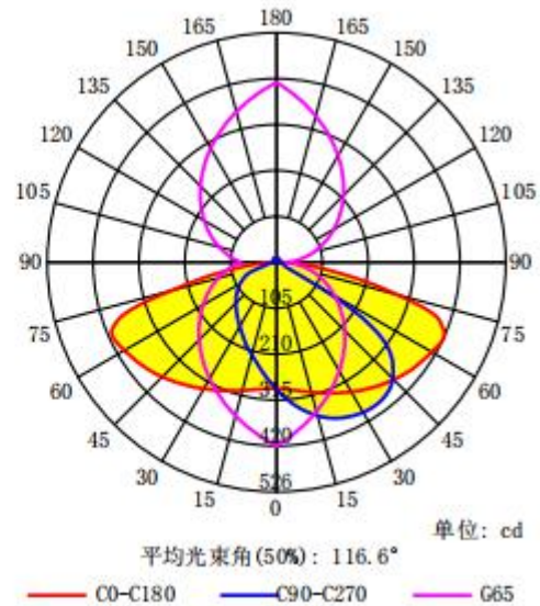
配光曲线
