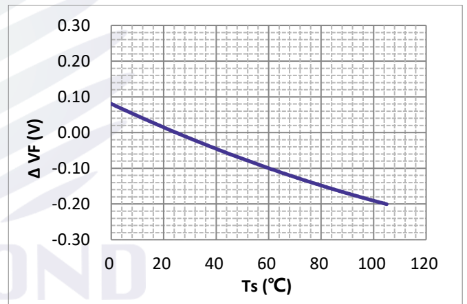
Forward voltage vs. T_s temperature 电压与温度曲线 ( I_F=800\text{mA} )
