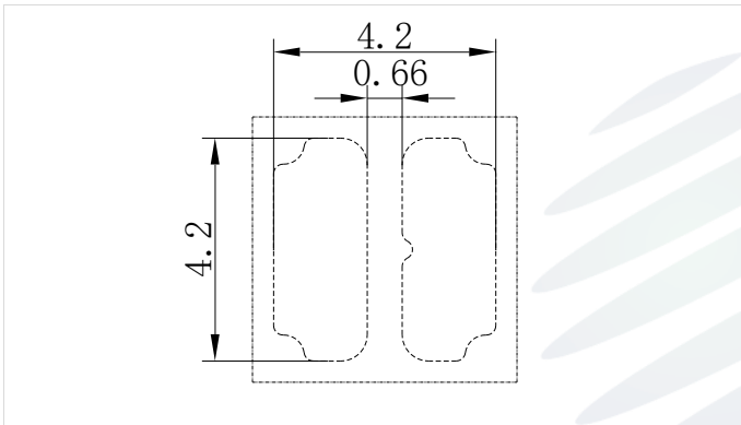
Bottom view 背面视图
